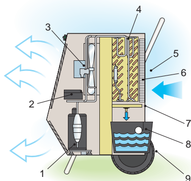
Figuur 1 Hoe het apparaat werkt: 1. Luchtdichtcompressor. 2. Controleinstrument. 3. Schroefvormige ventilator. 4. Condensor. 5. Luchtfilter. 6. Verdamer. 7. Slangfitting. 8. Vlotter. 9. Waterbak (niet in DH 80).
